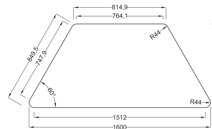
TAVOLO TRAPEZIO DA 160
